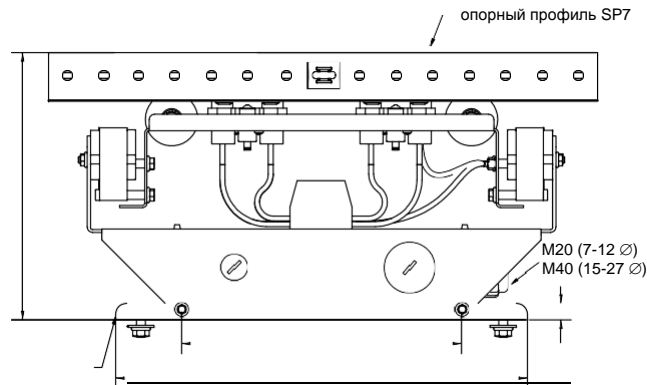
Опорный кронштейн PCT7-MB125 для токосъемной тележки
