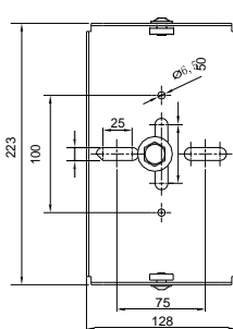
Кронштейн SP10-MB
