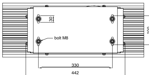
Опорный кронштейн РСТ10-MB125
