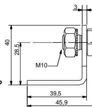
Клеммный соединитель C(J)-LC400 вид сбоку
