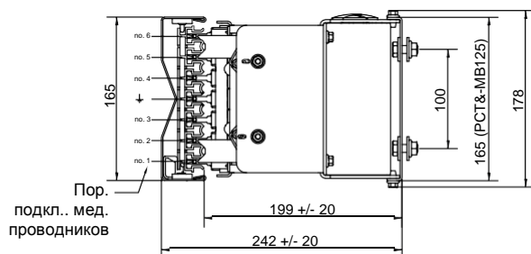
Опорный кронштейн PCT7-MB125 для токосъемной тележки
