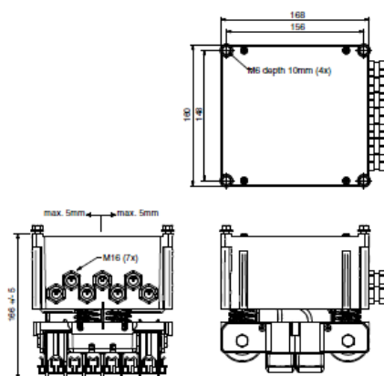
Токосъемник PCT7-7-70/NT
