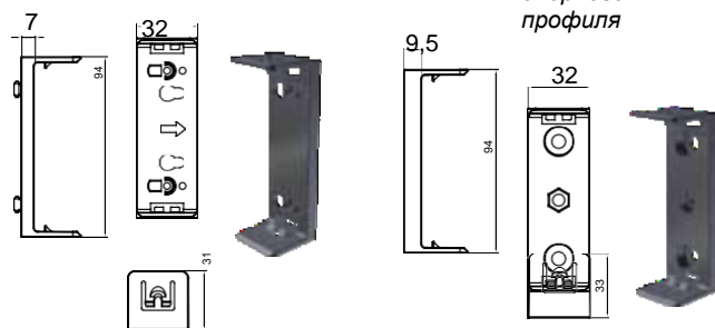
Опорный кронштейн PR4-MB (для установки без SP4)
